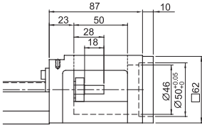
Motor Adaptor Flange F1
